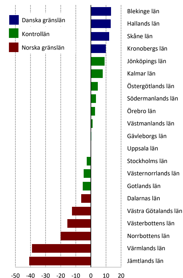
Figur 2: Förändring i försäljning till följd av begränsad gränshandel (DiD-analys)
